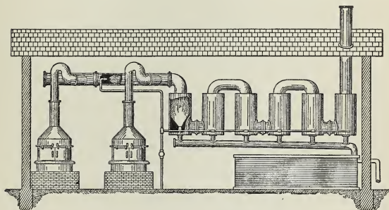
FIG. 20.—Condenser.
